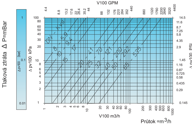
Diagram tlakové ztráty (pro medium voda)
