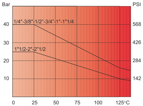
Diagram tlaku a teploty (Test prováděný vodou)
